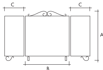
SALVACHISPAS S TRES CUERPOS
